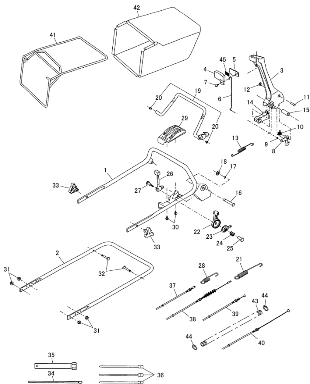
図4 ハンドル部
