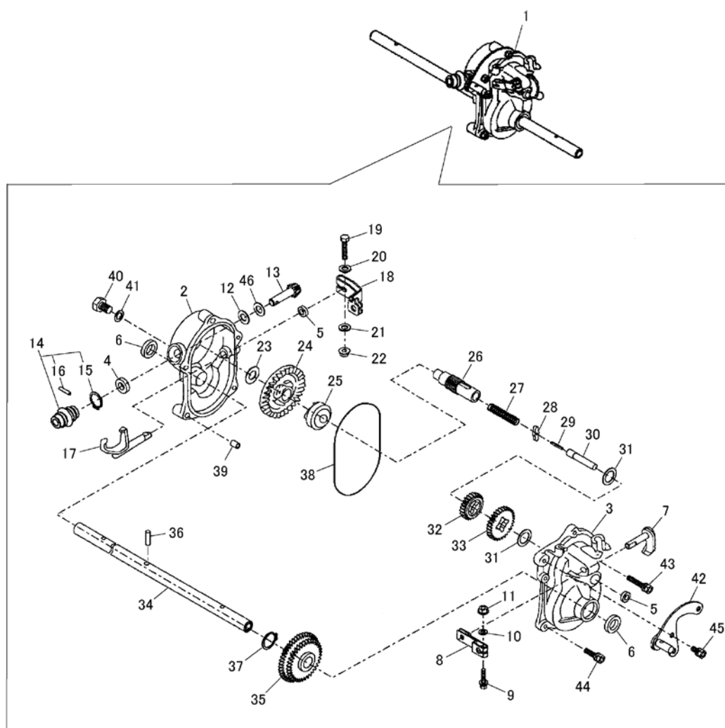
図1 ギヤケース
