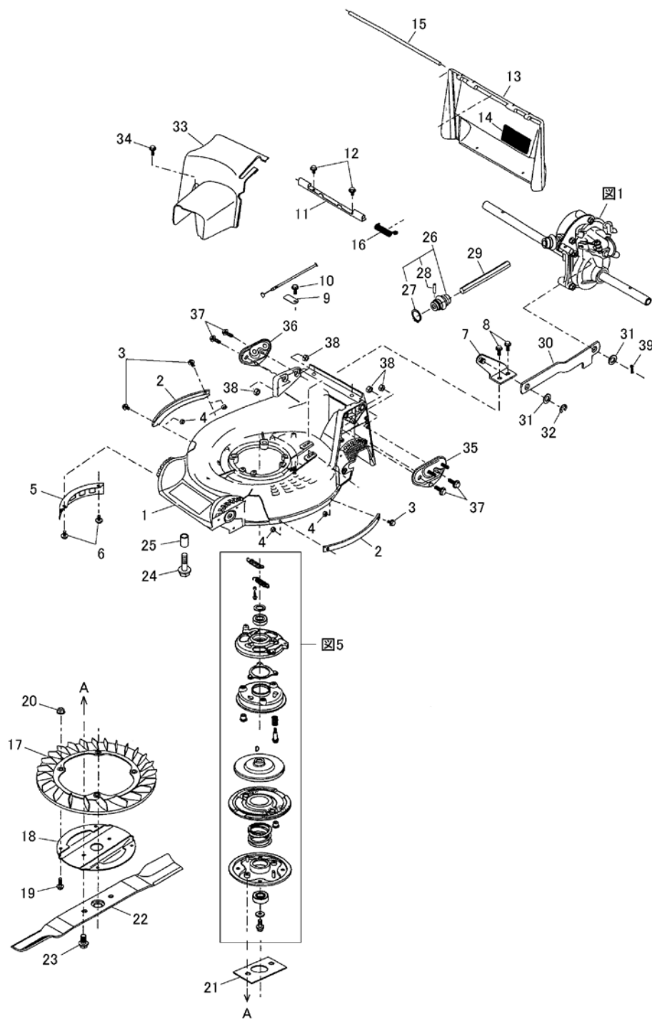
図3 刈取り部
